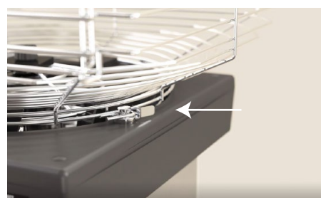
6. Acciona la pestaña de bloqueo.
