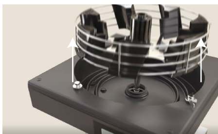
20. Extraire le panier inférieur.
