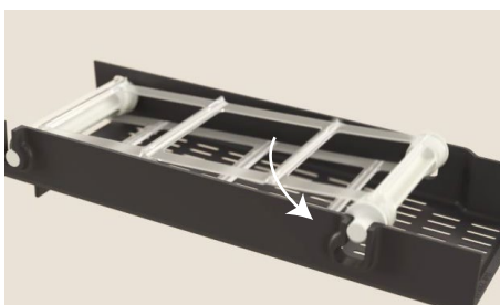
10. Fixer la raclette et l'introduire dans le bac Adapt.
